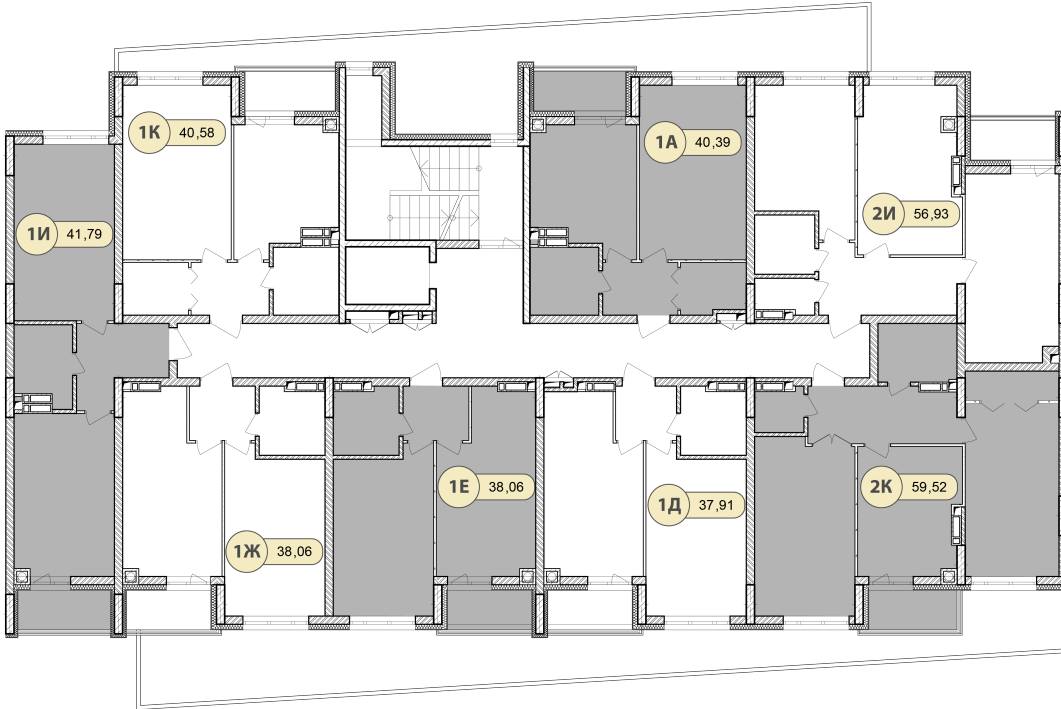
Типовий поверх
