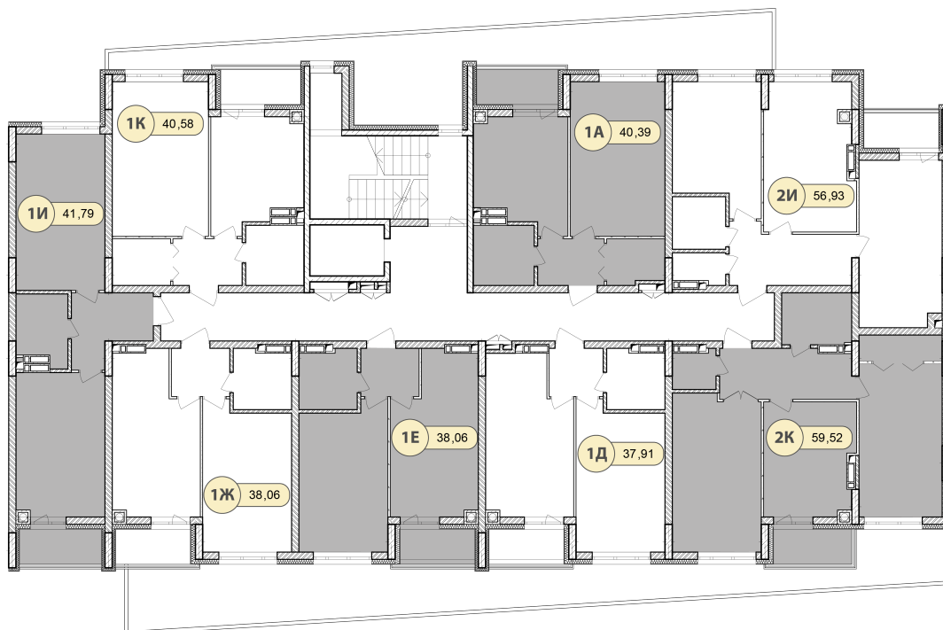
Типовий поверх
